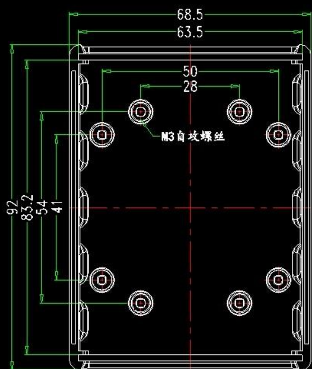
上壳内视图
