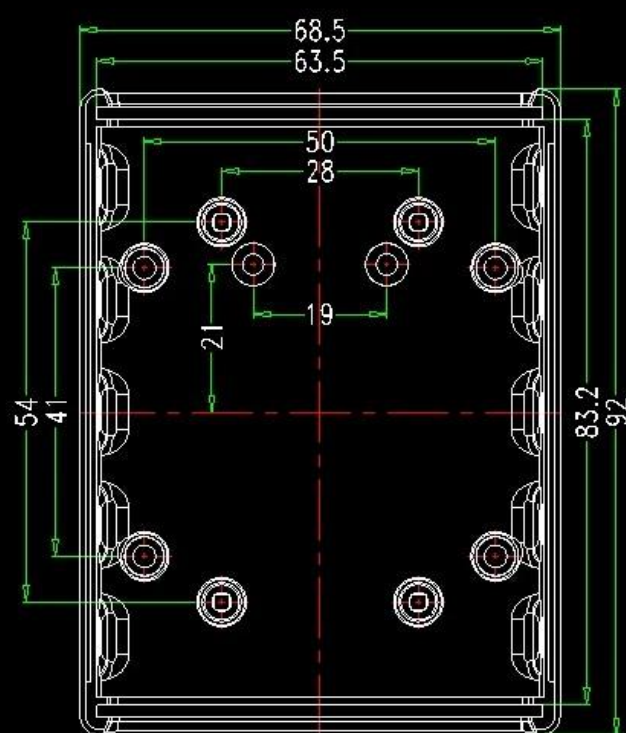
下壳内视图
