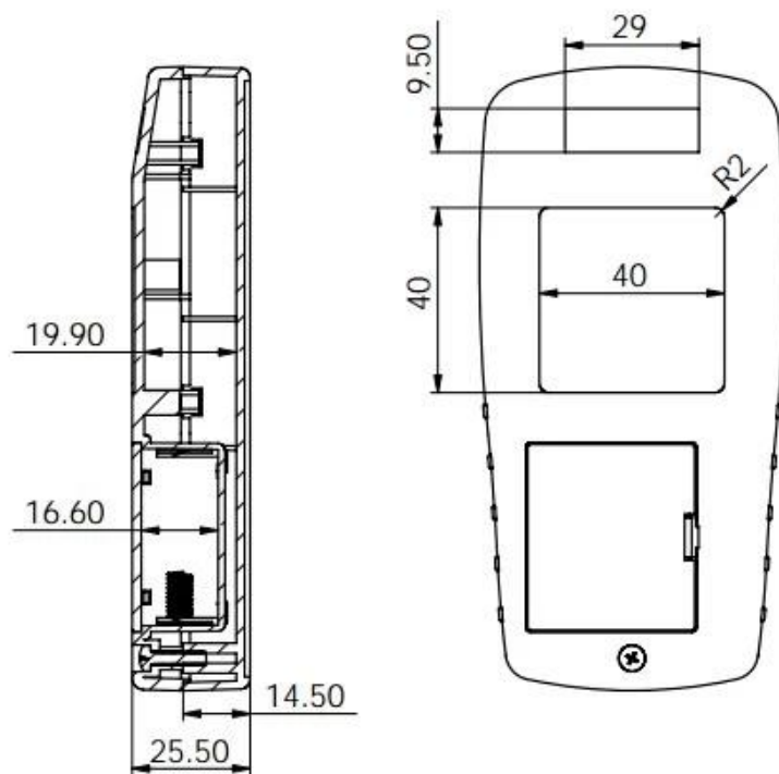
剖面 A-A
