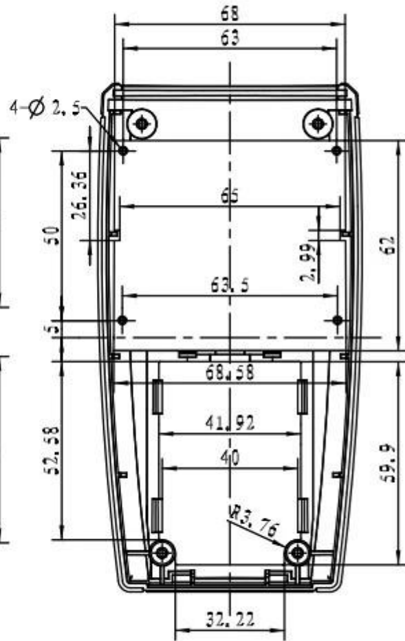
下壳线路板和电池仓尺寸
