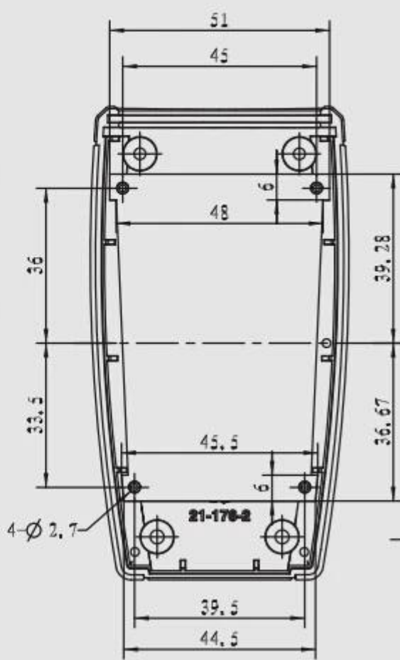
下壳线路板尺寸
