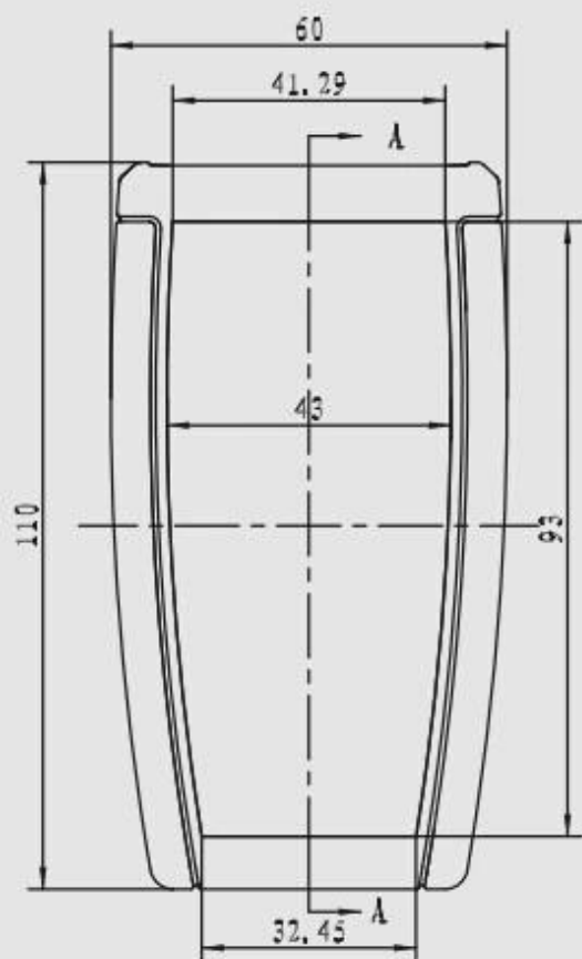
上盖线路板尺寸
