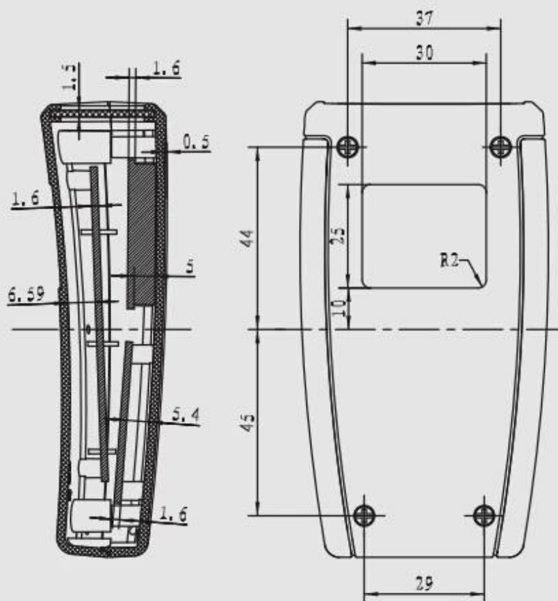
下壳线路板尺寸
