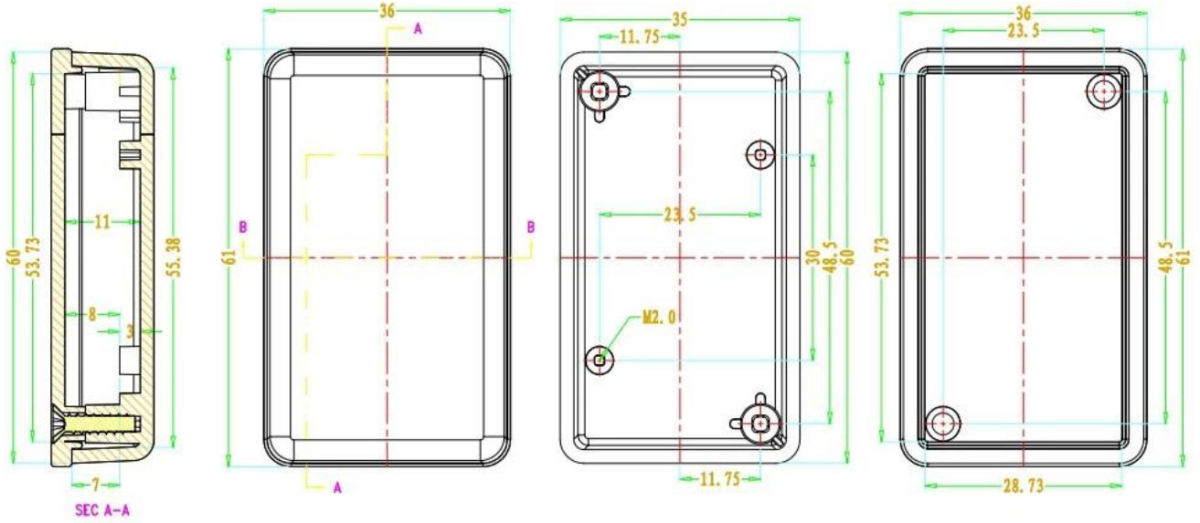
SEC A-A
