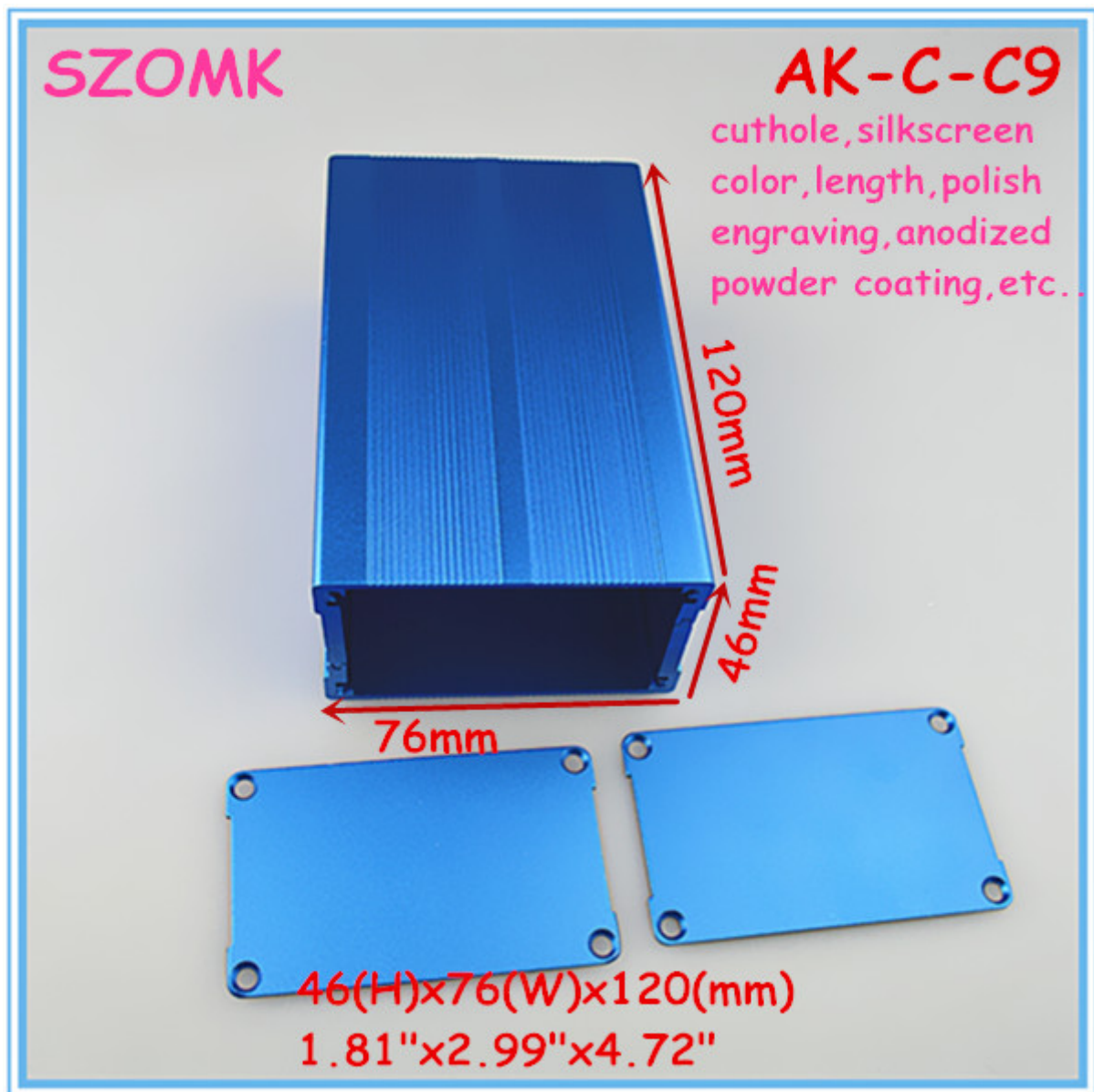
Dibujo de aluminio caja de extrusión para el módulo de sensor
