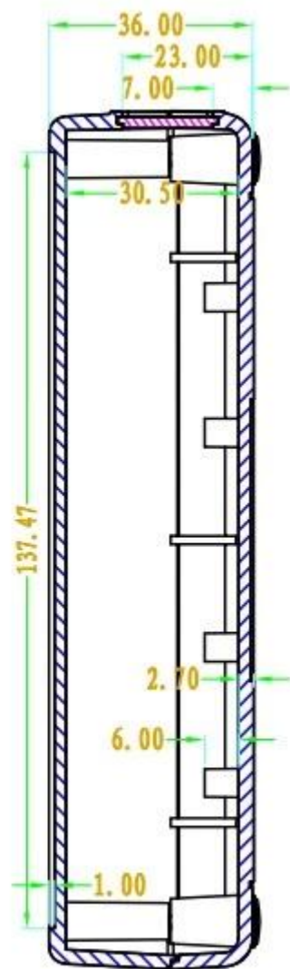
SEC A-A
