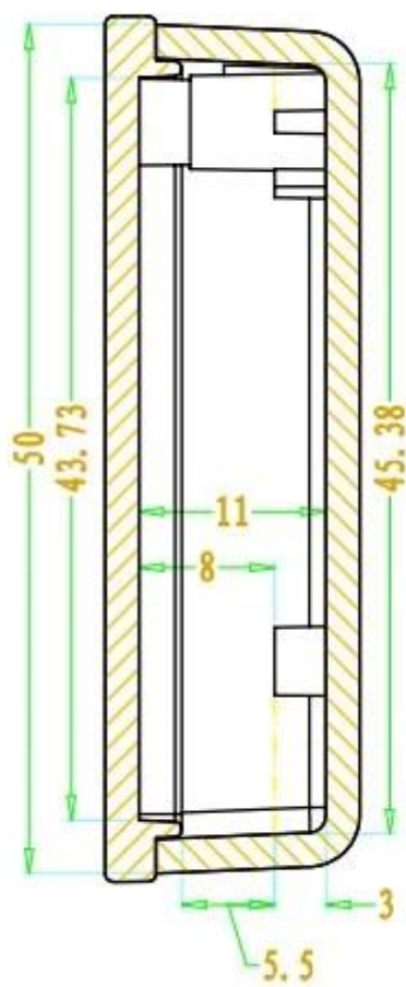
SEC A-A
