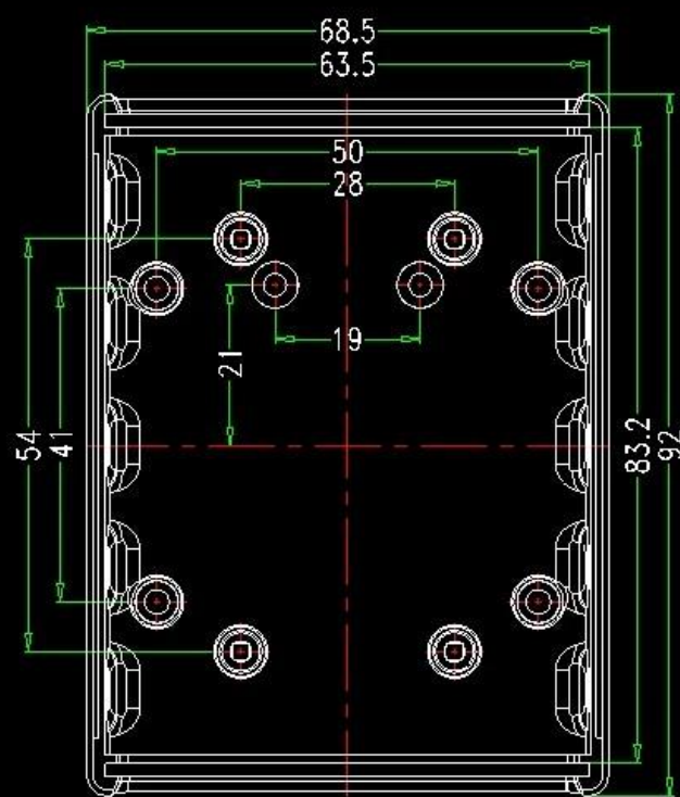
下壳内视图
