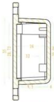
SEC A-A
