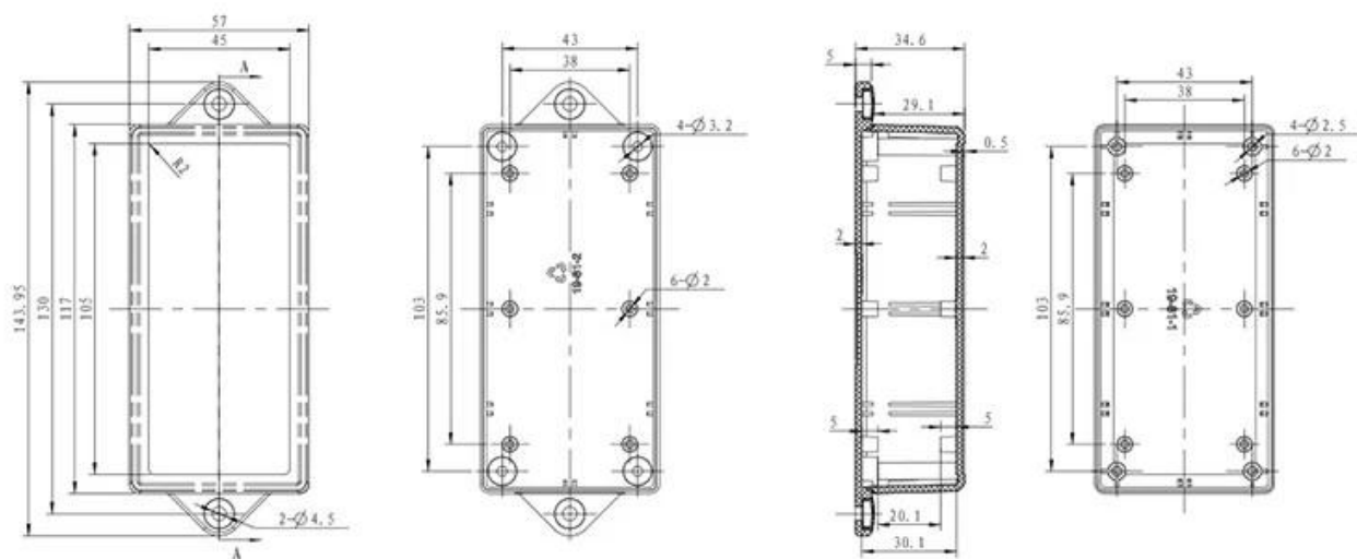
剖面 A-A
