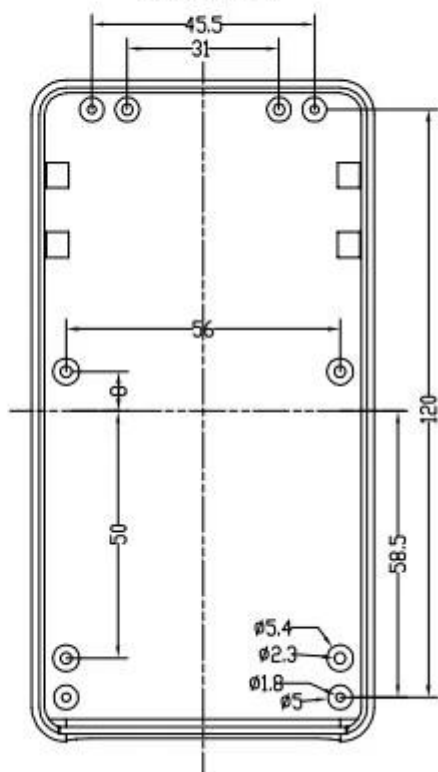
上盖底视图
