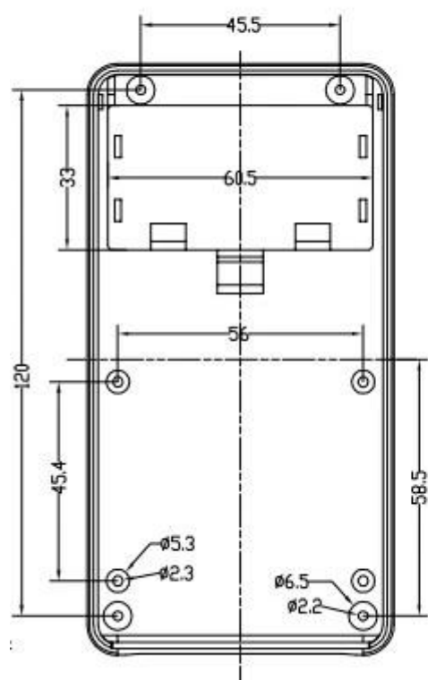
下盖正视图
