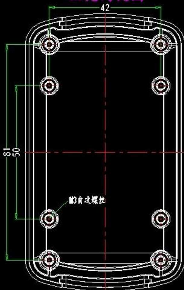
上壳内视图
