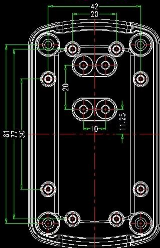
底壳内视图
