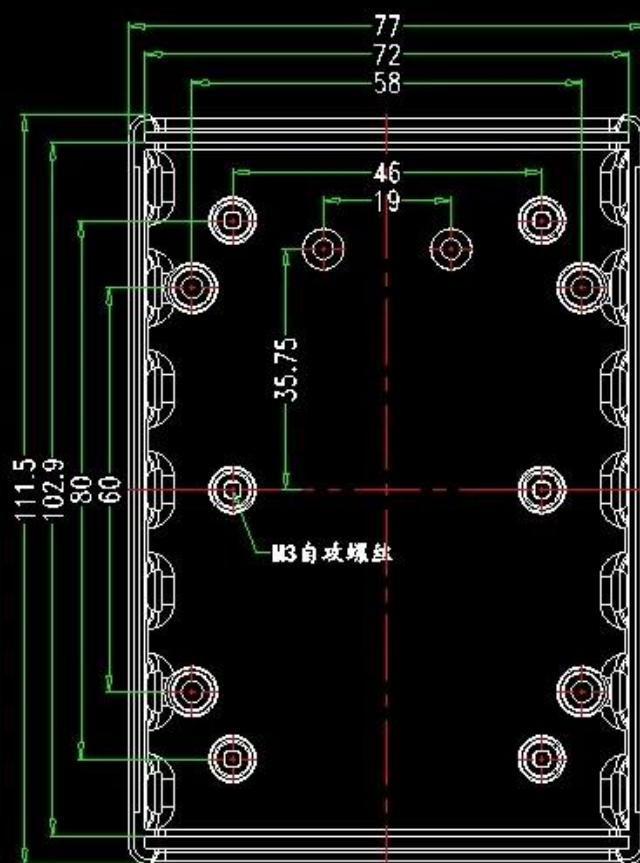
下壳内视图
