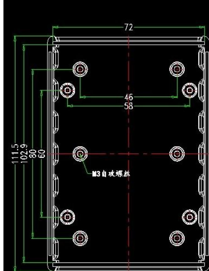
上壳内视图
