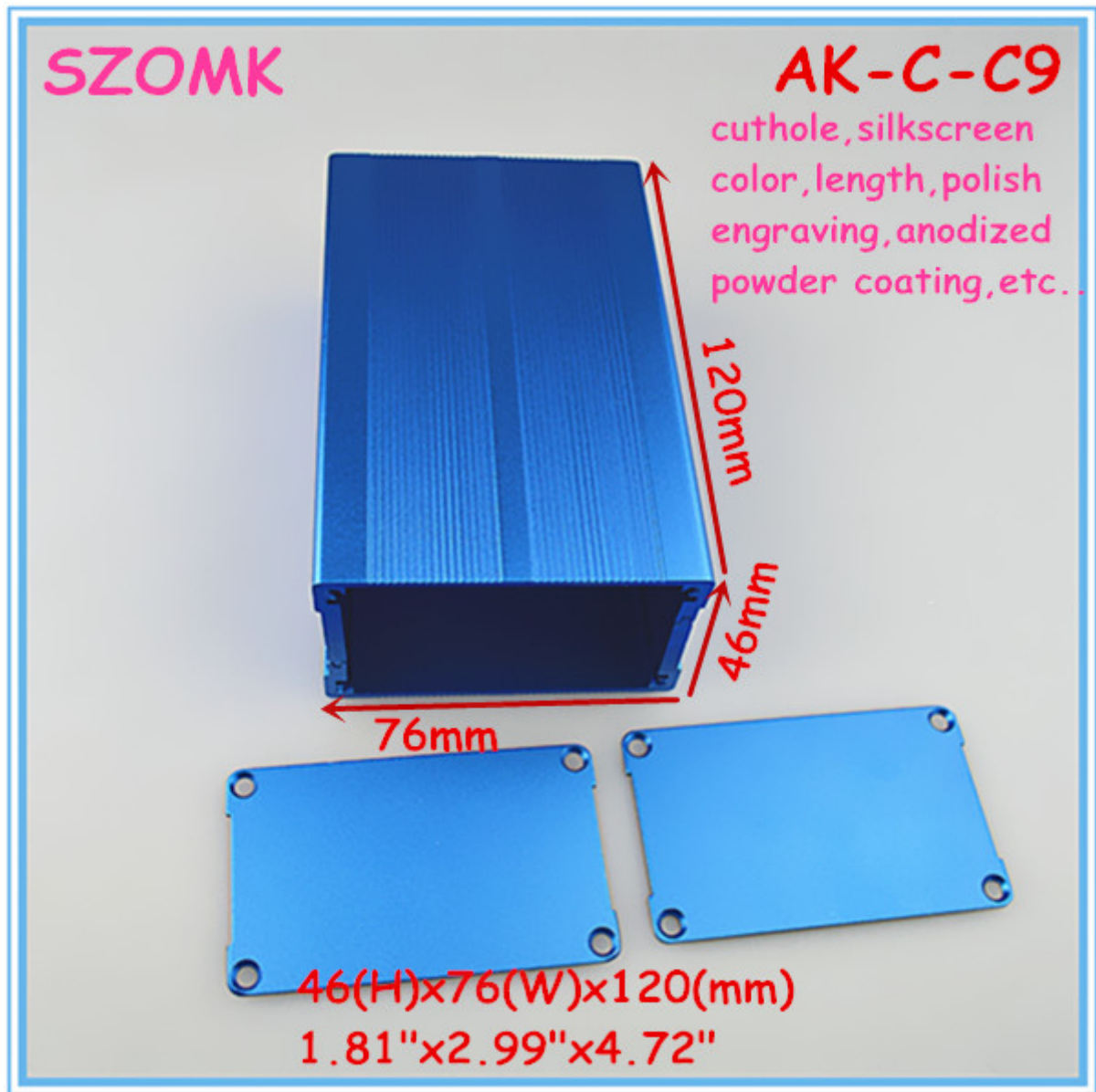
Tekening van aluminium behuizing extrusie voor sensormodule
