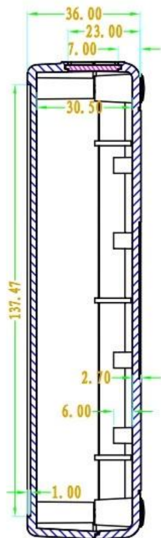
SEC A-A
