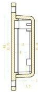
SEC A-A
