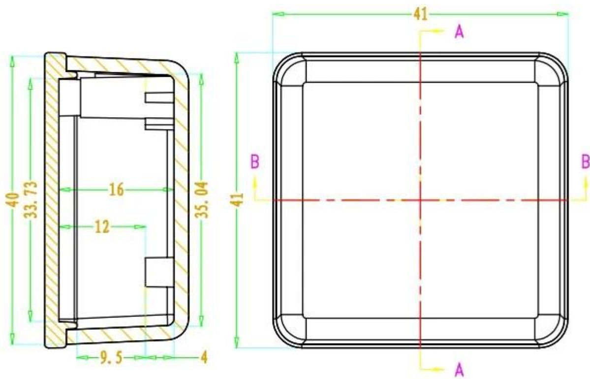
SEC A-A
