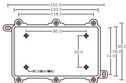
AK-BW-04 140*85*56mm
