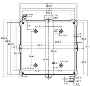
AK-BW-08 134*134*66mm
