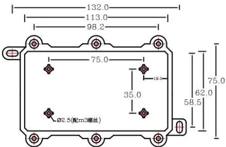
AK-BW-03 120*70*48mm
