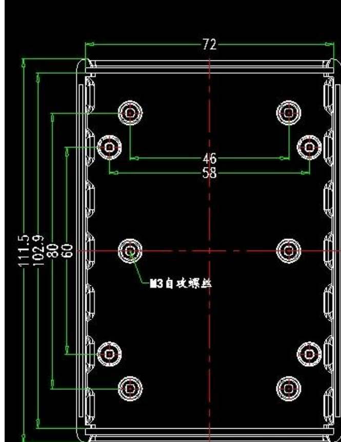
上壳内视图
