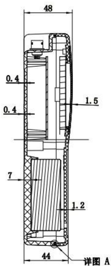
截面 A-A
