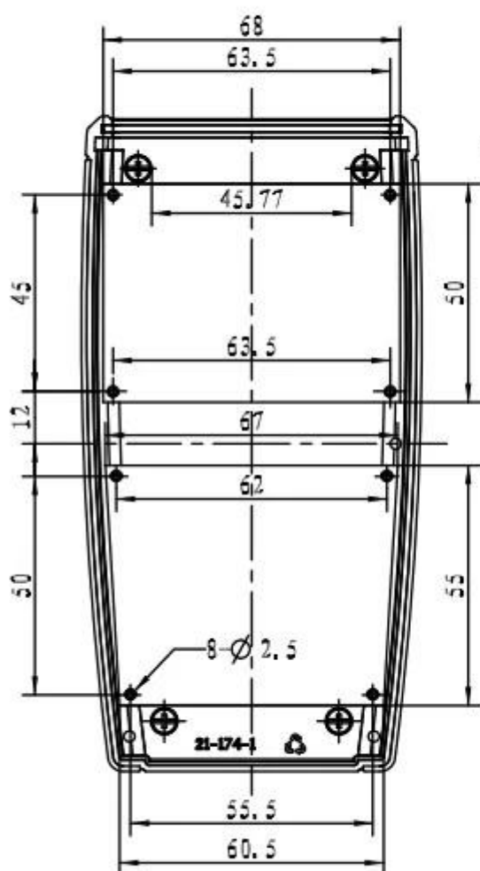
上蓋線路板尺寸
