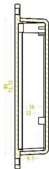
SEC A-A
