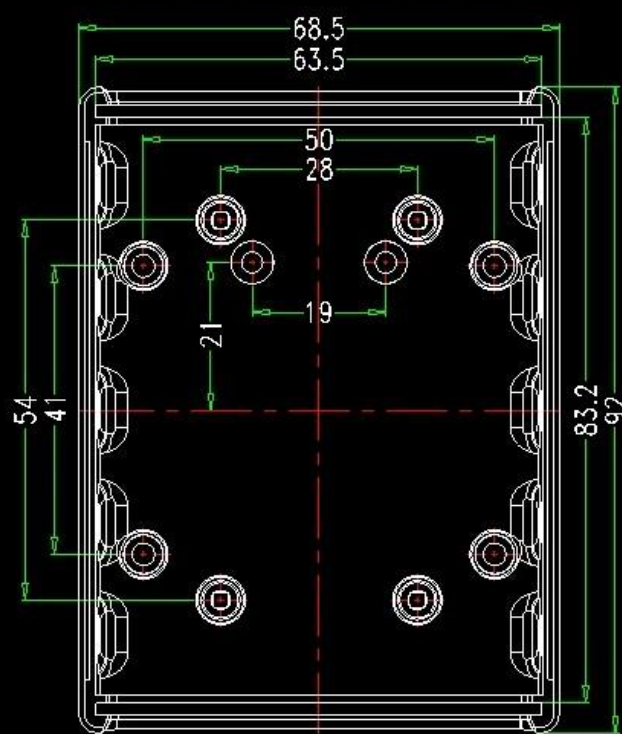
下壳内视图
